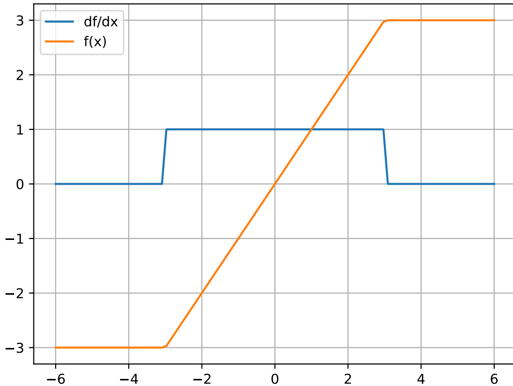
hard_tanh(x, lower_bound=-3, upper_bound=3)
