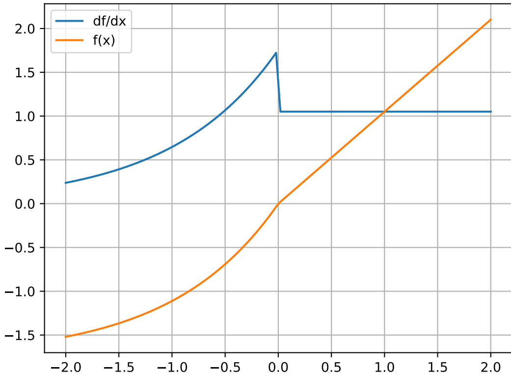
selu(x)
