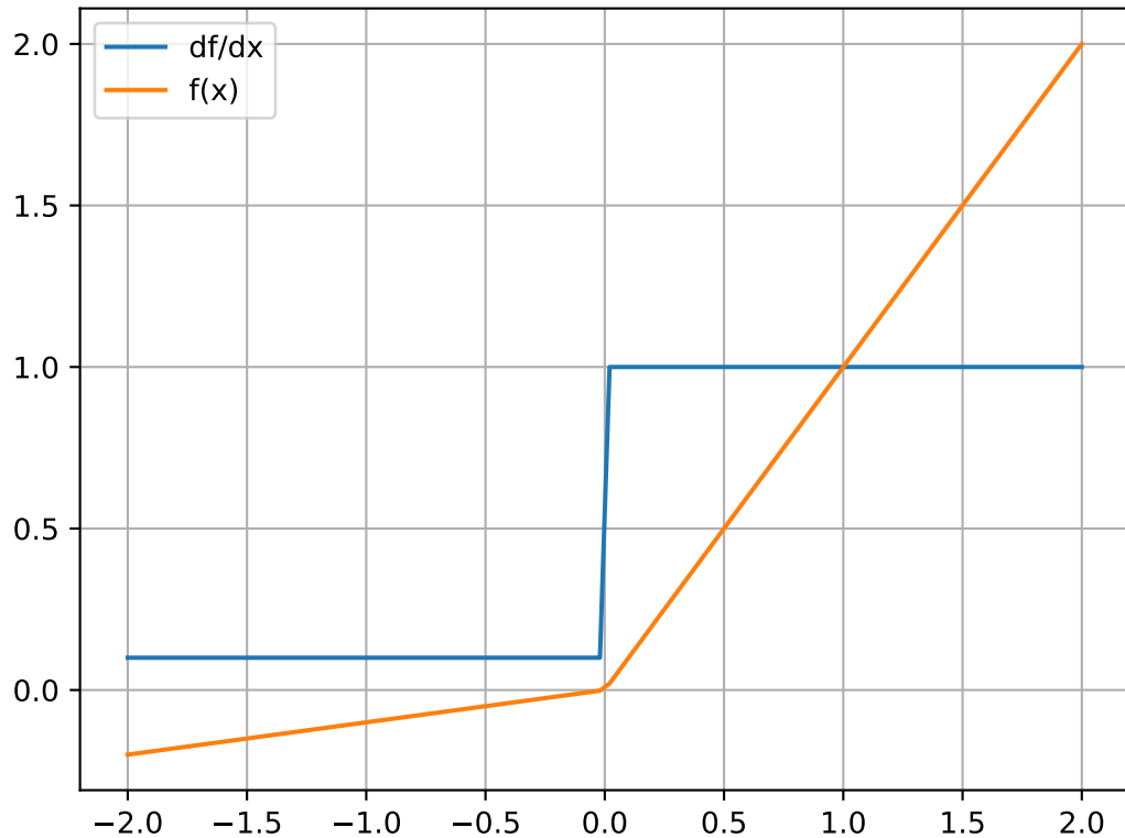
leaky_relu(x, slope=0.1)
