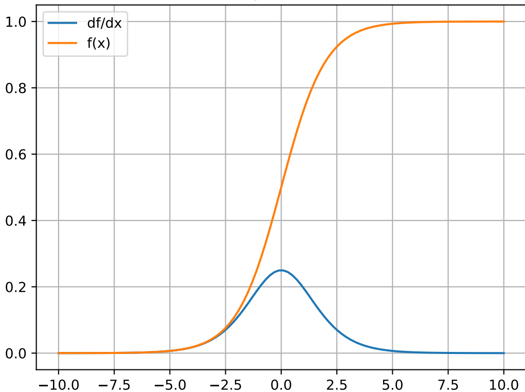
sigmoid(x)
